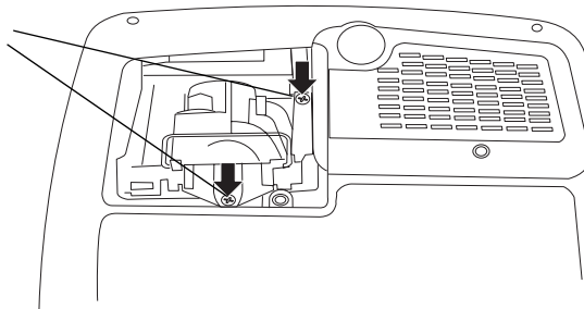
выкрутите винты на модуле лампы
