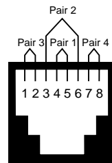
T568A
