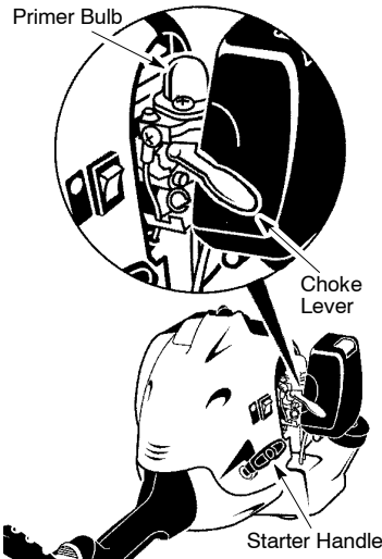
Primer Bulb
