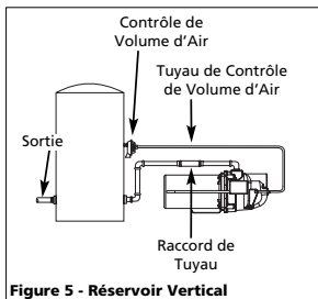
Figure 5 - Réservoir Vertical
