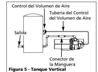
Figura 5 - Tanque Vertical
