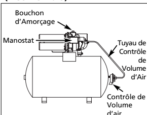
Figure 4 - Réservoir Horizontal
