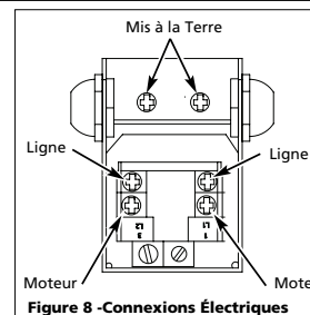
Figure 8 - Connexions Électriques
