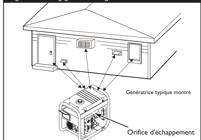
Figure 10 — Dégagement de la génératrice
