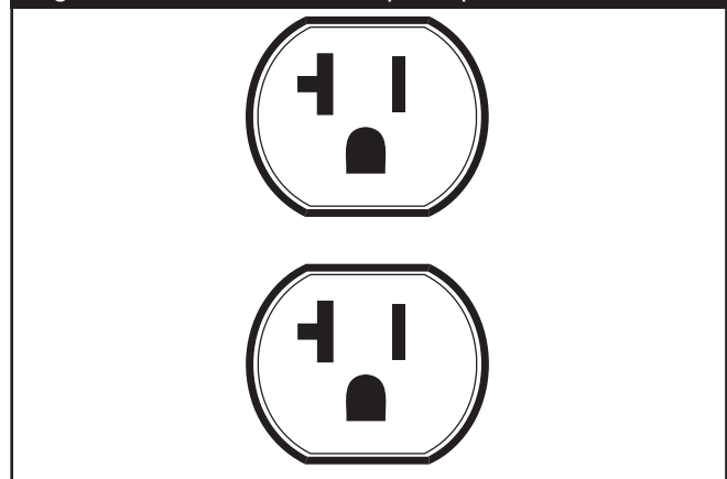
Figura 20 — 120 Volt AC, 20 Amp Receptáculo Doble
