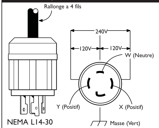
Figure 12 – Prise à Verrouillage de 120/240 Volts c.a., 30 Ampères
