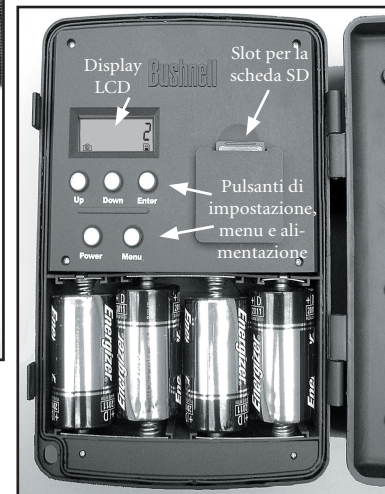
Dettaglio Pulsanti e Display
