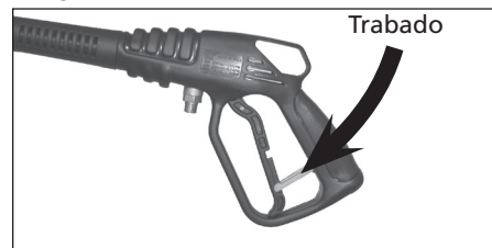
Figura 8 - Gatillo trabado
