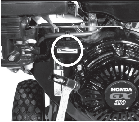
Figura 10 - Obturador
