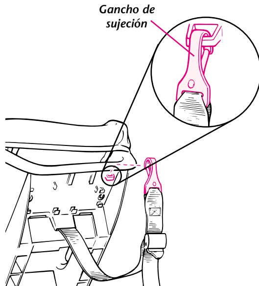
Respaldo del asiento para el automóvil
